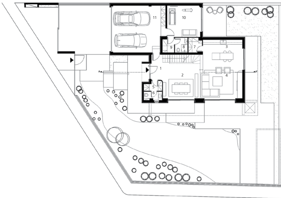
κάτοψη ισογείου
