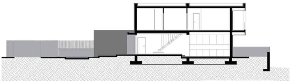
τομή α-α'
